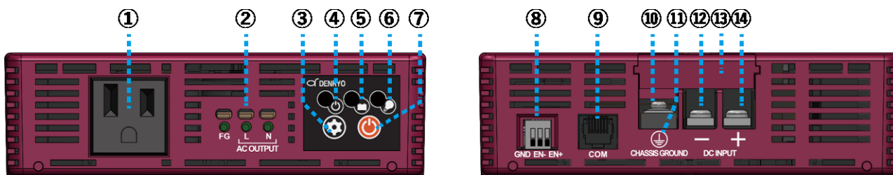
前面パネル
